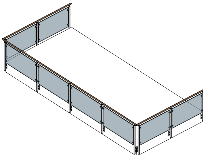
BALUSTRADA STALOWA DOCZOŁOWA TYP 1A PORECZ OKRĄGŁA + SZKŁO LB
