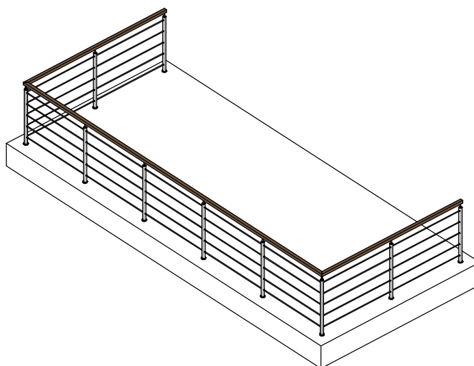
BALUSTRADA STALOWA TYP 1 + PRĘTY LB
