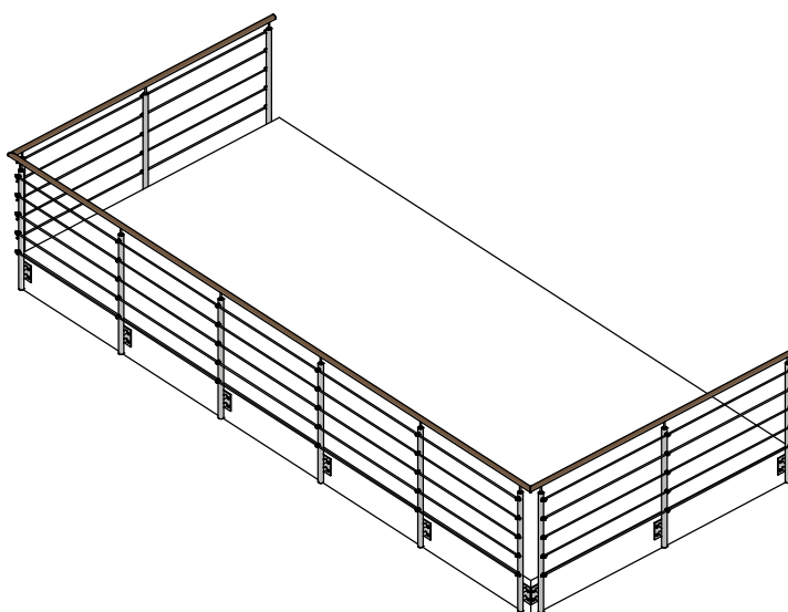
BALUSTRADA STALOWA TYP 3 DOCZOŁOWA PORECZ OKRĄGŁA + PRĘTY LB
