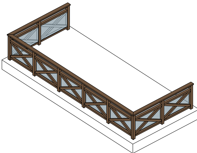
BALUSTRADA DREWNIANA KRZYŻULCOWA TYP 3B + SZKŁO LB
