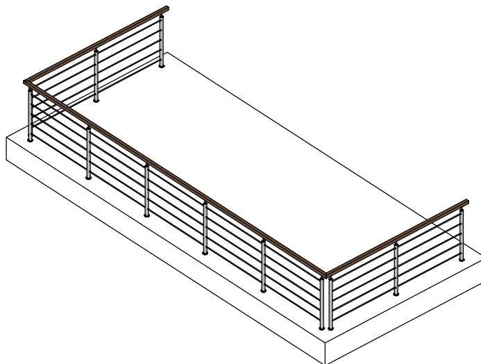
BALUSTRADA STALOWA TYP 1A + PRĘTY LB
