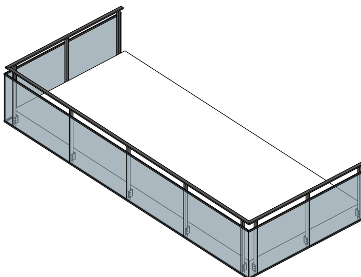
BALUSTARADA SAMONOŚNA SZKLANA TYP 6 SZKLANA DOCZOŁOWA MO LB
