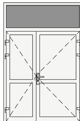
DRZWI WEW ALU-PCV PEŁNE 2X2 ASYMETRYCZNE + NAŚWITLĘ GÓRNE
