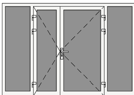
DRZWI WEW ALU-PCV PRZESZKLONE 2X ASYMETRYCZNE + NAŚWITLĘ BOCZNE
