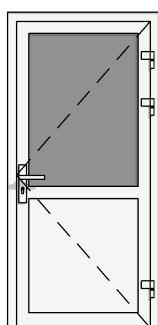
DRZWI WEW ALU-PCV PEŁNE+PRZESZKLONE 1X2 100x210
