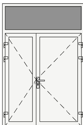
DRZWI WEW ALU-PCV PEŁNE 2X ASYMETRYCZNE + NAŚWITLĘ GÓRNE
