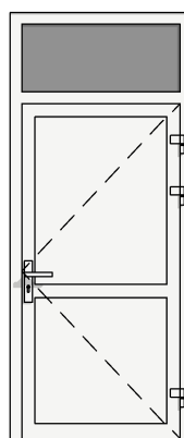
DRZWI WEW ALU-PCV PEŁNE 1X2 + NAŚWITŁE GÓRNE
