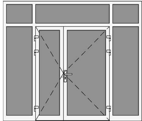
DRZWI WEW ALU-PCV PRZESZKLONE 2X ASYMETRYCZNE + NASWIECLE GÓRNE I BOCZNE
