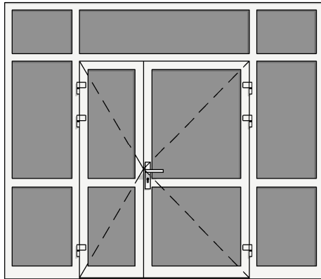
DRZWI WEW ALU-PCV PRZESZKLONE 2X2 ASYMETRYCZNE + NASWIECLE GÓRNE I BOCZNE
