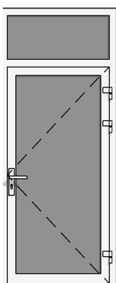
DRZWI WEW ALU-PCV PRZESZKLONE 1X+NAŚWITŁE GÓRNE 110x260 (205)
