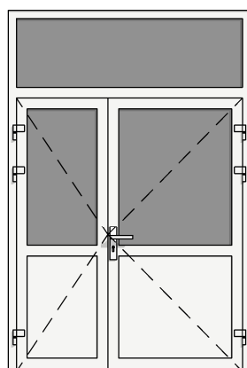
DRZWI WEW ALU-PCV PEŁNE+PRZESZKLONE 2X2 ASYMETRYCZNE + NAŚWITLĘ GÓRNE
