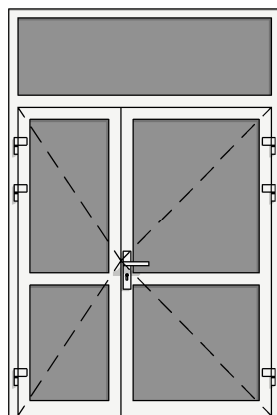
DRZWI WEW ALU-PCV PRZESZKLONE 2X2 ASYMETRYCZNE + NAŚWITLĘ GÓRNE
