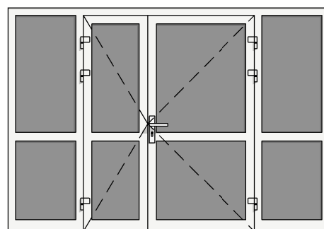
DRZWI WEW ALU-PCV PRZESZKLONE 2X2 ASYMETRYCZNE + NAŚWITLĘ BOCZNE
