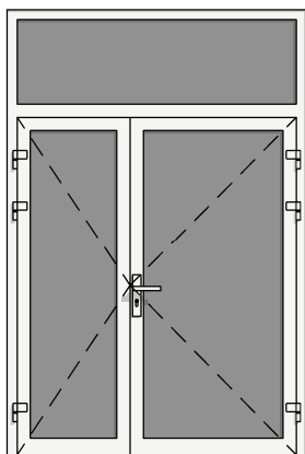
DRZWI WEW ALU-PCV PRZESZKLONE 2X ASYMETRYCZNE + NAŚWITLĘ GÓRNE
