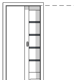
DW TYP 1 PRZESUWNE 1X CHOWANE W ŚCIANĘ 90 Z PODCIĘCIEM
