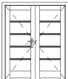
DW TYP 1 2X 2X80 Z PODCIĘCIEM
