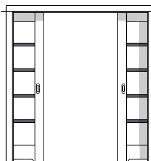
DW TYP 1 PRZESUWNE 2X CHOWANE W ŚCIANĘ 2x90 Z PODCIĘCIEM
