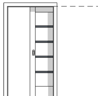
DW TYP 1 PRZESUWNE 1X CHOWANE W ŚCIANĘ 100
