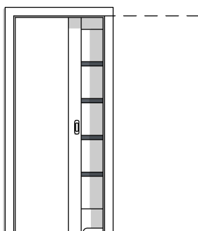
DW TYP 1 PRZESUWNE 1X CHOWANE W ŚCIANĘ 80 Z PODCIĘCIEM
