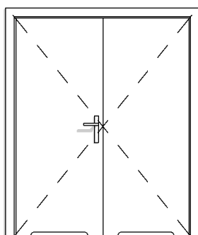
DW TYP 3 2X 2X80 Z PODCIĘCIEM
