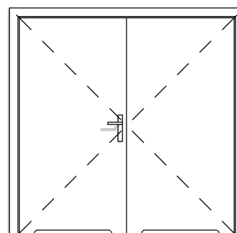
DW TYP 3 2X 2X100 Z PODCIĘCIEM
