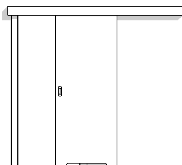
DW TYP 3 PRZESUWNE NAKLADANE 1X 80 Z PODCIĘCIEM
