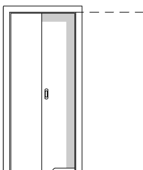
DW TYP 3 PRZESUWNE 1X CHOWANE W ŚCIANĘ 80
