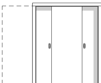
DW TYP 3 PRZESUWNE 2X CHOWANE W ŚCIANĘ 2x80
