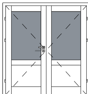
DW TYP 4A 2X PRZYLGOWE 2X90 PRZESZKLENIE GÓRA
