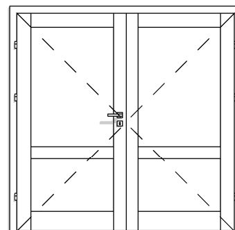
DW TYP 4A 2X PRZYLGOWE 2X100 PEŁNE
