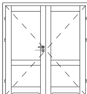
DW TYP 4A 2X PRZYLGOWE 2X90 PEŁNE Z PODCIĘCIEM
