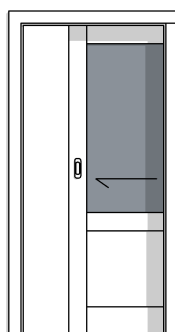
DW TYP 4A PRZESUWNE 1X CHOWANE W ŚCIANĘ 90 PRZESZKLONE GÓRA
