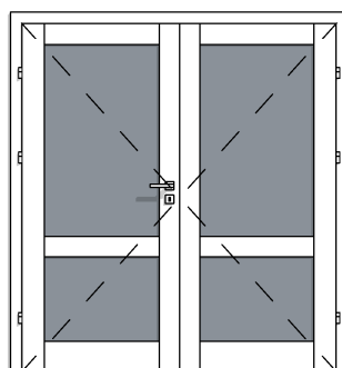
DW TYP 4A 2X PRZYLGOWE 2X90 PRZESZKLENIE GÓRA+DÓŁ
