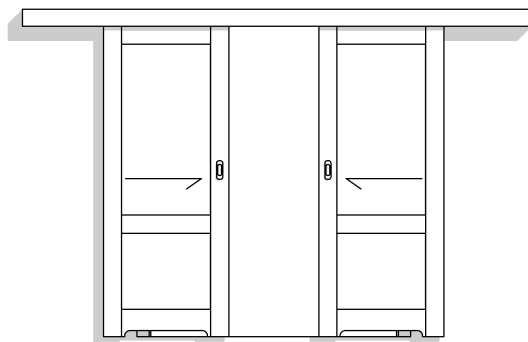
DW TYP 4A 2X PRZESUWNE NAKLADANE 2X80 PEŁNE Z PODCIĘCIEM
