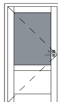
DW TYP 4A 1X PRZYLGOWE 100 PRZESZKLENIE GÓRA
