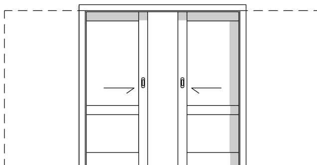
DW TYP 4A PRZESUWNE 2X CHOWANE W ŚCIANĘ 2x100 PEŁNE
