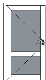
DW TYP 4A 1X PRZYLGOWE 100 PRZESZKLENIE GÓRA+DÓŁ
