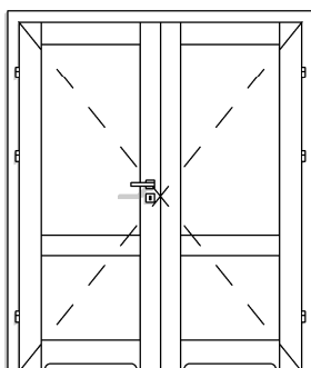
DW TYP 4A 2X PRZYLGOWE 2X80 PEŁNE Z PODCIĘCIEM
