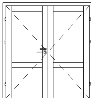
DW TYP 4A 2X PRZYLGOWE 2X90 PEŁNE
