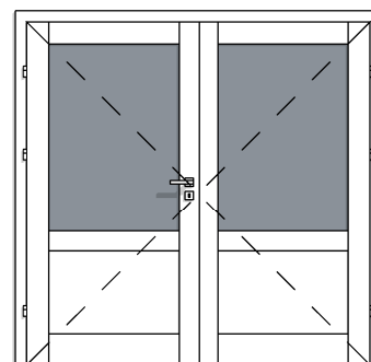
DW TYP 4A 2X PRZYLGOWE 2X100 PRZESZKLENIE GÓRA
