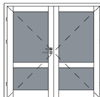
DW TYP 4A 2X PRZYLGOWE 2X100 PRZESZKLENIE GÓRA+DÓŁ
