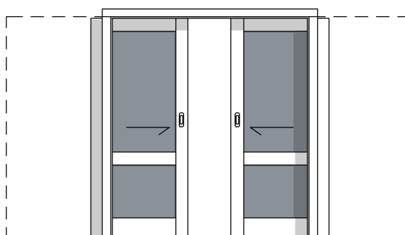
DW TYP 4A PRZESUWNE 2X CHOWANE W ŚCIANĘ 2x90 PRZESZKLENIE GÓRA+DÓŁ
