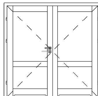
DW TYP 4A 2X PRZYLGOWE 2X100 PEŁNE Z PODCIĘCIEM
