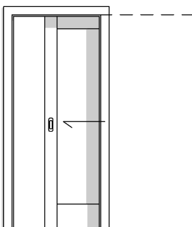
DW TYP 5A PRZESUWNE 1X CHOWANE W ŚCIANĘ 80
