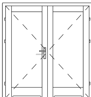
DW TYP 5A 2X PRZYLGOWE 2x90 Z PODCIĘCIEM
