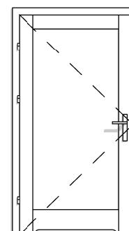
DW TYP 5A 1X PRZYLGOWE 100_Z PODCIĘCIEM
