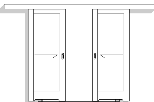
DW TYP 5A 2X PRZESUWNE NAKŁADANE 80 Z PODCIECIEM
