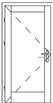
DW TYP 5A 1X PRZYLGOWE 90
