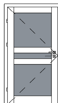
DW TYP 7A 1X PRZYLGOWE 100 PRZESZKLENIE CAŁKOWITE
