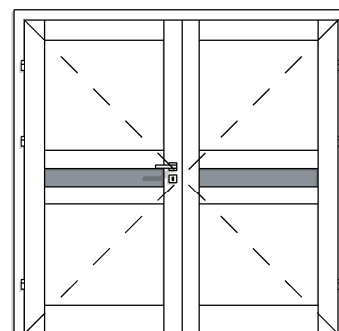
DW TYP 7A 2X PRZYLGOWE 2X100 PRZESZKLENIE ŚRODEK
