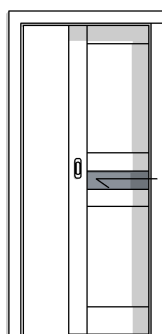
DW TYP 7A PRZESUWNE 1X CHOWANE W ŚCIANĘ 80 PRZESZKLONE ŚRODEK
