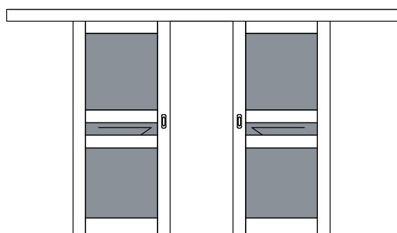
DW TYP 7A 2X PRZESUWNE NAKLADANE 2X90 PRZESZKLENIE CAŁKOWITE
