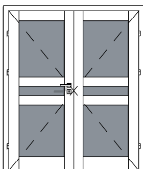
DW TYP 7A 2X PRZYLGOWE 2X80 PRZESZKLENIE CAŁKOWITE
