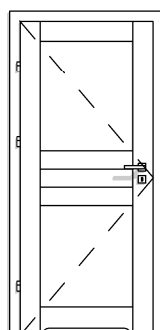
DW TYP 7A 1X PRZYLGOWE 80 PEŁNE Z PODCIĘCIEM
