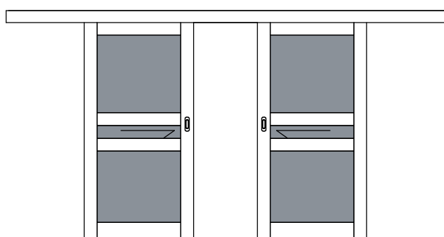
DW TYP 7A 2X PRZESUWNE NAKLADANE
