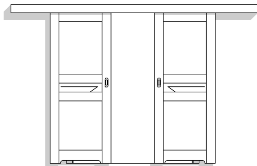
DW TYP 7A 2X PRZESUWNE NAKLADANE 2X80 PEŁNE Z PODCIĘCIEM
