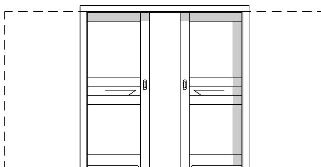
DW TYP 7A PRZESUWNE 2X CHOWANE W ŚCIANĘ 2x100 PEŁNE Z PODCIĘCIEM
