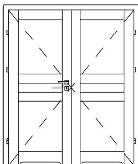
DW TYP 7A 2X PRZYLGOWE 2X80 PEŁNE Z PODCIĘCIEM
