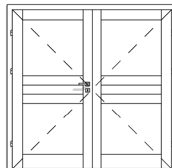
DW TYP 7A 2X PRZYLGOWE 2X100 PEŁNE
