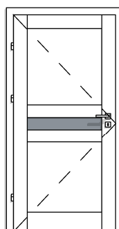
DW TYP 7A 1X PRZYLGOWE 90 PRZESZKLENIE ŚRODEK
