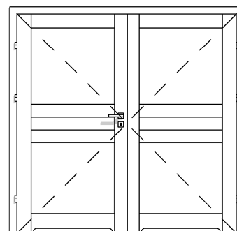
DW TYP 7A 2X PRZYLGOWE 2X100 PEŁNE Z PODCIĘCIEM
