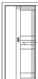
DW TYP 7A PRZESUWNE 1X CHOWANE W ŚCIANĘ 80 PEŁNE Z PODCIĘCIEM
