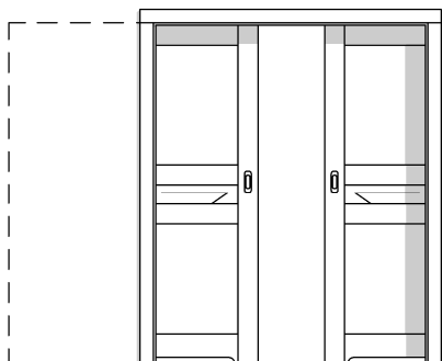
DW TYP 7A PRZESUWNE 2X CHOWANE W ŚCIANĘ 2x80 PEŁNE Z PODCIĘCIEM
