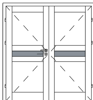
DW TYP 7A 2X PRZYLGOWE 2X90 PRZESZKLENIE ŚRODEK
