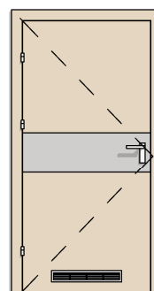
DW TYP 8 1X BEZPRZYLGOWE 90 PEŁNE + BLACHA ŚRODKOWA + KRATKA
