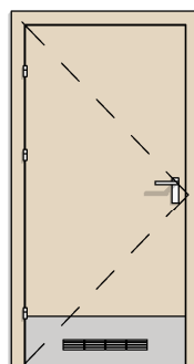
DW TYP 8 1X BEZPRZYLGOWE 90 PEŁNE + BLACHA DOLNA + KRATKA
