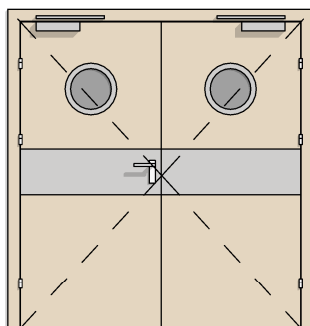
DW TYP 8 2X BEZPRZYLGOWE 90+90 BULAJ + BLACHA ŚRODKOWA + SAMOZAMYKACZ 2X 2
