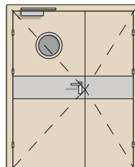
DW TYP 8 2X BEZPRZYLGOWE 90+60 BULAJ + PEŁNE + BLACHA DOLNA + SAMOZAMYKACZ 1X
