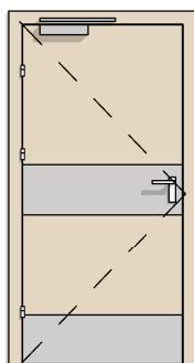
DW TYP 8 1X BEZPRZYLGOWE 90 PEŁNE + BLACHA I ŚRODKOWA + SAMOZAMYKACZ
