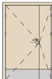
DW TYP 8 2X BEZPRZYLGOWE 90+30 PEŁNE + BLACHA DOLNA
