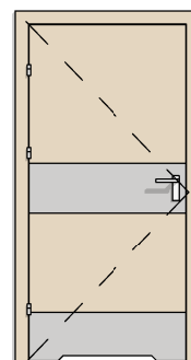
DW TYP 8 1X BEZPRZYLGOWE 90 PEŁNE + BLACHA DOLNA I ŚRODKOWA + PODCIĘCIE
