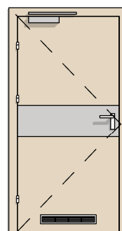
DW TYP 8 1X BEZPRZYLGOWE 90 PEŁNE + BLACHA ŚRODKOWA + KRATKA + SAMOZAMYKACZ
