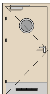
DW TYP 8 1X BEZPRZYLGOWE 90 BULAJ + BLACHA DOLNA + KRATKA + SAMOZAMYKACZ
