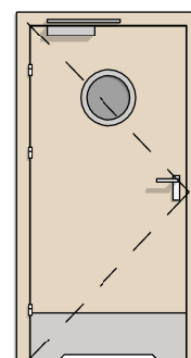
DW TYP 8 1X BEZPRZYLGOWE 90 BULAJ + BLACHA DOLNA + PODCIĘCIE + SAMOZAMYKACZ
