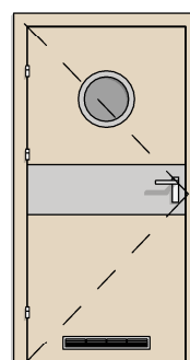
DW TYP 8 1X BEZPRZYLGOWE 90 BULAJ + BLACHA ŚRODKOWA + KRATKA + SAMOZAMYKACZ
