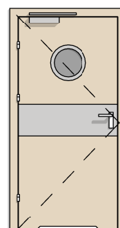
DW TYP 8 1X BEZPRZYLGOWE 90 BULAJ + BLACHA ŚRODKOWA + PODCIĘCIE + SAMOZAMYKACZ
