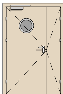
DW TYP 8 2X BEZPRZYLGOWE 90+30 BULAJ 1X + SAMOZAMYKACZ 1X
