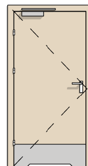
DW TYP 8 1X BEZPRZYLGOWE 90 PEŁNE + BLACHA DOLNA + PODCIĘCIE + SAMOZAMYKACZ
