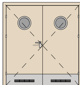
DW TYP 8 2X BEZPRZYLGOWE 90+90 BULAJ + BLACHA DOLNA + KRATKA
