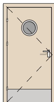
DW TYP 8 1X BEZPRZYLGOWE 90 BULAJ + BLACHA DOLNA
