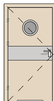
DW TYP 8 1X BEZPRZYLGOWE 90 BULAJ + BLACHA ŚRODKOWA + PODCIĘCIE
