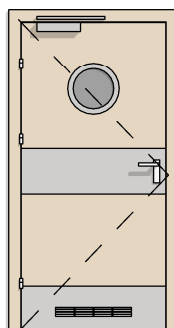
DW TYP 8 1X BEZPRZYLGOWE 90 BULAJ + BLACHA DOLNA I ŚRODKOWA + KRATKA + SAMOZAMYKACZ
