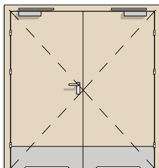
DW TYP 8 2X BEZPRZYLGOWE 90+90 PEŁNE + PODCIĘCIE + BLACHA DOLNA + SAMOZAMYKACZ 2X
