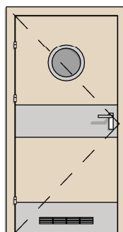
DW TYP 8 1X BEZPRZYLGOWE 90 BULAJ + BLACHA DOLNA I ŚRODKOWA + KRATKA
