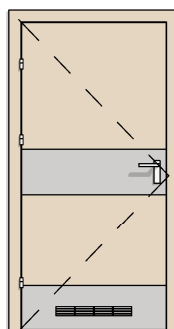
DW TYP 8 1X BEZPRZYLGOWE 90 PEŁNE + BLACHA DOLNA I ŚRODKOWA + KRATKA
