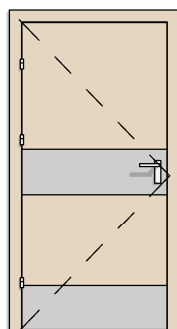
DW TYP 8 1X BEZPRZYLGOWE 90 PEŁNE + BLACHA I ŚRODKOWA
