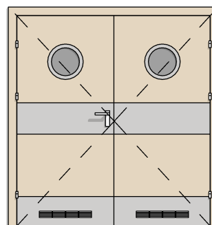
DW TYP 8 2X BEZPRZYLGOWE 90+90 BULAJ + BLACHA DOLNA/SRODKOWA + KRATKA
