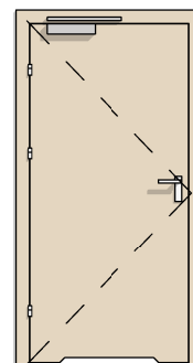
DW TYP 8 1X BEZPRZYLGOWE 90 PEŁNE + PODCIĘCIE + SAMOZAMYKACZ
