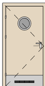
DW TYP 8 1X BEZPRZYLGOWE 90 BULAJ + BLACHA DOLNA + KRATKA
