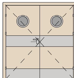
DW TYP 8 2X BEZPRZYLGOWE 90+90 BULAJ + BLACHA DOLNA/SRODKOWA
