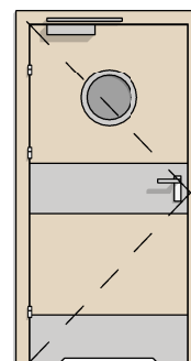
DW TYP 8 1X BEZPRZYLGOWE 90 BULAJ + BLACHA DOLNA I ŚRODKOWA + PODCIĘCIE + SAMOZAMYKACZ
