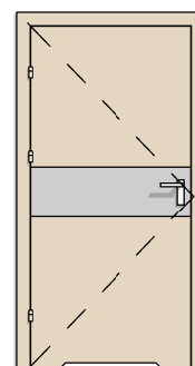
DW TYP 8 1X BEZPRZYLGOWE 90 PEŁNE + BLACHA ŚRODKOWA + PODCIĘCIE
