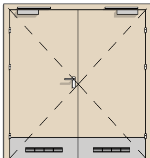
DW TYP 8 2X BEZPRZYLGOWE 90+90 PEŁNE + PODCIĘCIE + BLACHA DOLNA + KRATKA + SAMOZAMYKACZ 2X
