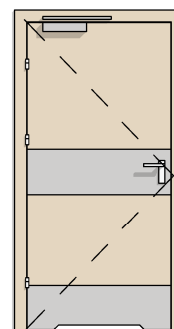
DW TYP 8 1X BEZPRZYLGOWE 90 PEŁNE + BLACHA DOLNA I ŚRODKOWA + PODCIĘCIE + SAMOZAMYKACZ
