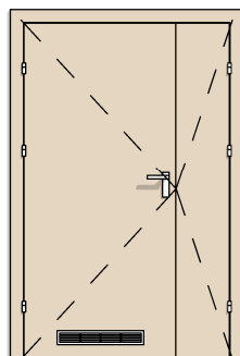
DW TYP 8 2X BEZPRZYLGOWE 90+30 PEŁNE + KRATKA 1X
