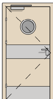
DW TYP 8 1X BEZPRZYLGOWE 90 BULAJ + BLACHA DOLNA I ŚRODKOWA + SAMOZAMYKACZ
