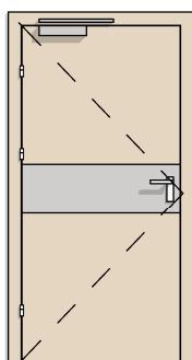
DW TYP 8 1X BEZPRZYLGOWE 90 PEŁNE + BLACHA ŚRODKOWA + SAMOZAMYKACZ
