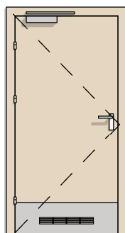
DW TYP 8 1X BEZPRZYLGOWE 90 PEŁNE + BLACHA DOLNA + KRATKA + SAMOZAMYKACZ
