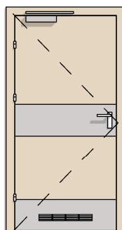
DW TYP 8 1X BEZPRZYLGOWE 90 PEŁNE + BLACHA DOLNA I ŚRODKOWA + KRATKA + SAMOZAMYKACZ
