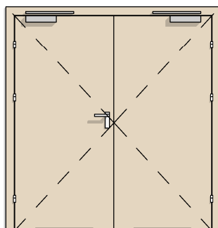
DW TYP 8 2X BEZPRZYLGOWE 90+90 PEŁNE + PODCIĘCIE + SAMOZAMYKACZ
