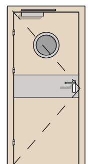
DW TYP 8 1X BEZPRZYLGOWE 80 BULAJ + BLACHA ŚRODKOWA + SAMOZAMYKACZ
