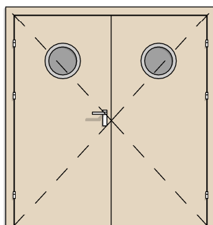
DW TYP 8 2X BEZPRZYLGOWE 90+90 BULAJ
