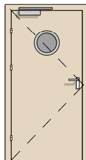
DW TYP 8 1X BEZPRZYLGOWE 90 BULAJ + SAMOZAMYKACZ
