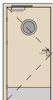
DW TYP 8 1X BEZPRZYLGOWE 90 BULAJ + BLACHA DOLNA + SAMOZAMYKACZ
