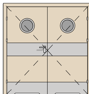
DW TYP 8 2X BEZPRZYLGOWE 90+90 BULAJ + BLACHA DOLNA/ŚRODKOWA + PODCIĘCIE
