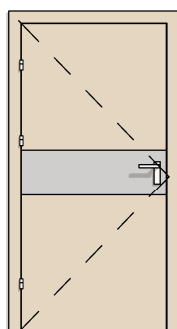
DW TYP 8 1X BEZPRZYLGOWE 90 PEŁNE + BLACHA ŚRODKOWA
