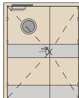
DW TYP 8 2X BEZPRZYLGOWE 90+60 BULAJ + PEŁNE + BLACHA DOLNA/ŚRODKOWA + SAMOZAMYKACZ 1X
