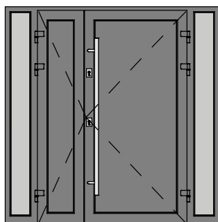
2X_PCV ENTRANCE DOOR TYPE 1 + 2X_NB
