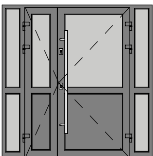
2X_PCV ENTRANCE DOOR TYPE 6A + 2X_NB
