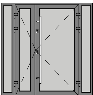
2X_PCV ENTRANCE DOOR TYPE 2 + 2X_NB
