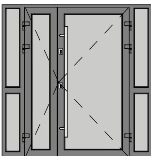
2X_PCV ENTRANCE DOOR TYPE 2A + 2X_NB
