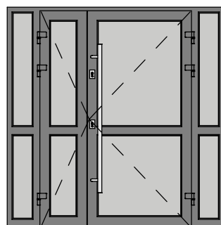
2X_PCV ENTRANCE DOOR TYPE 7A + 2X_NB
