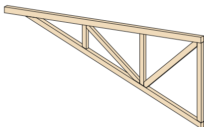
KRATOWNICA JEDNOSTRONNA TYP 1A 3X
