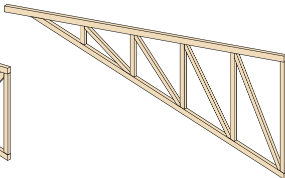
KRATOWNICA JEDNOSTRONNA TYP 1B 5X
