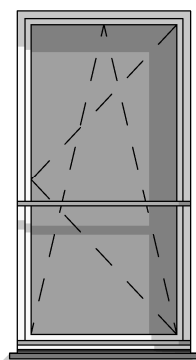
OKNO BALKONOWE PARAPET 1X + BALUSTRADA_SZKLANA WEW_2025 100X230 BALUSTRADA SZKLANA POZIOM
