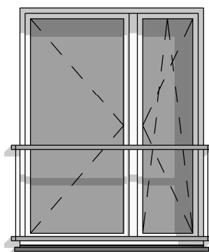
OKNO BALKONOWE PARAPET 2X1 + BALUSTRADA PROSTOKĄTNA_2025 180X230 BALUSTRADA SZKLANA
