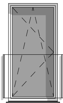
OKNO BALKONOWE PARAPET 1X + BALUSTRADA_2025 100X230 BALUSTRADA SZKŁO LISTWY
