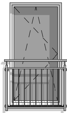
OKNO BALKONOWE PARAPET 1X + BALUSTRADA_NIERDZEWNA 2025 100X230 BALUSTRADA NIERDZEWKA SZCZ WEW PION
