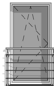
OKNO BALKONOWE PARAPET 1X + BALUSTRADA_NIERDZEWNA 2025 100X230 BALUSTRADA NIERDZEWKA SZCZ NAKŁ
