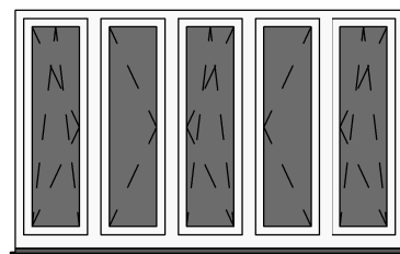
OKNO 5X SYMETRYCZNE 2026 240X150
