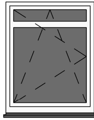
OKNO 1X SKRZYDŁO 1X2 2026 120x150
