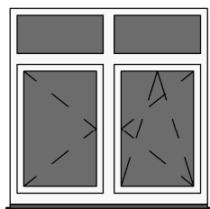
OKNO 2X2 O+W SYMETRYCZNE 2026 180 (120)x150
