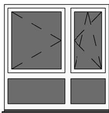
OKNO 2X2 W+O ASYMETRYCZNE 2026 150x150
