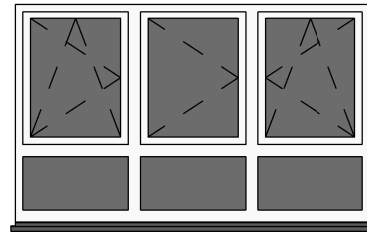
OKNO 3X2 W+O SYMETRYCZNE 2026 240X150
