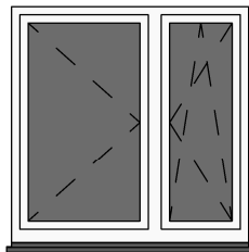
OKNO 2X ASYMETRYCZNE 2026 150(90)X150
