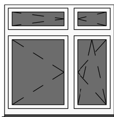
OKNO 2X2 ASYMETRYCZNE 2026 150(90)x150
