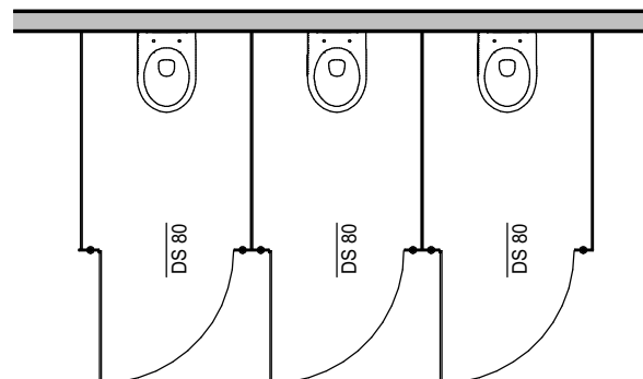
KABINY SANITARNE 3X TYP 3 GEBERIT ICON
